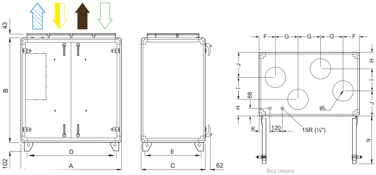
Вид сверху
