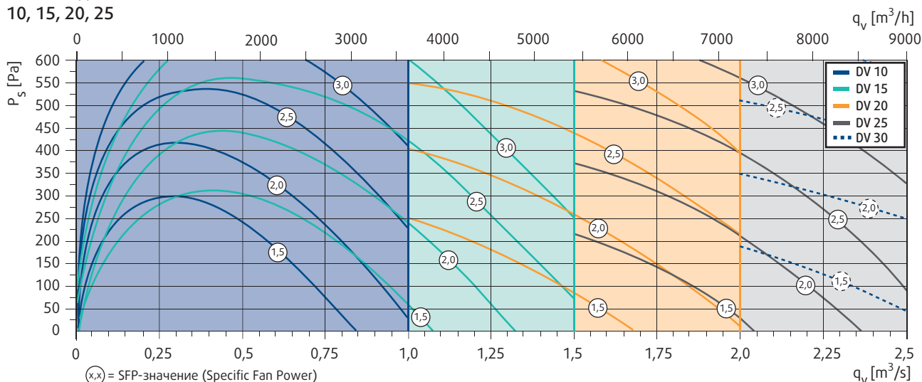
Рабочий диапазон 10, 15, 20, 25
