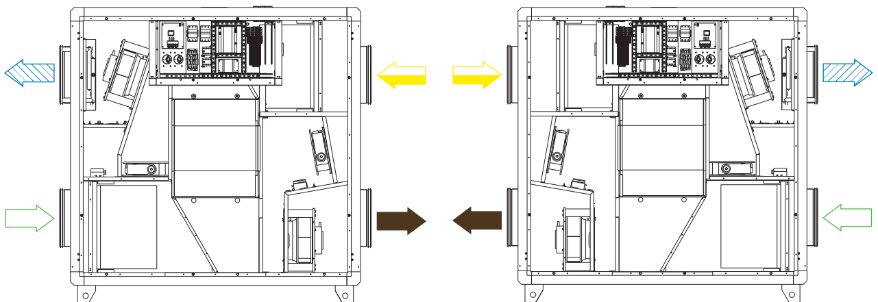
Левосторонний агрегат
